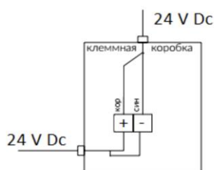
Схема подключения к сети постоянного тока 24 В DC
